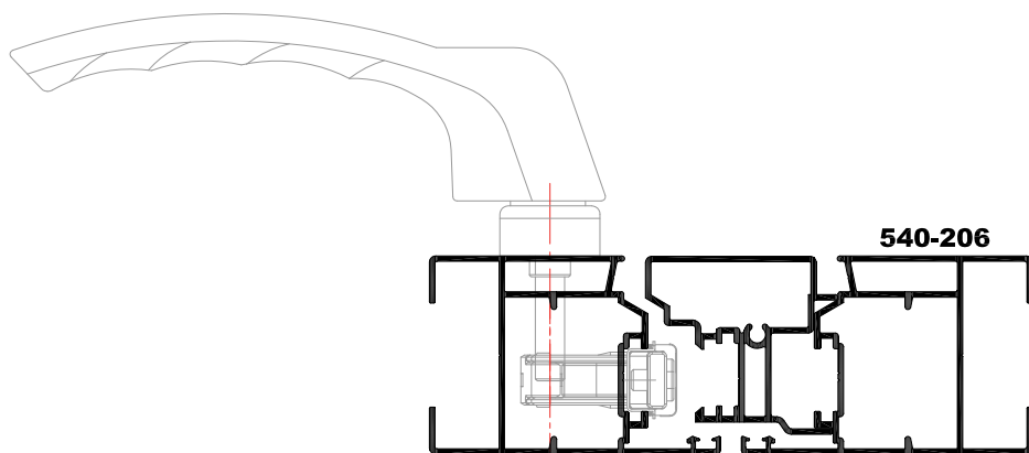
ΠΟΜΟΛΟ ΚΑΡΕ HANDLE WITH SQUARE PIN
